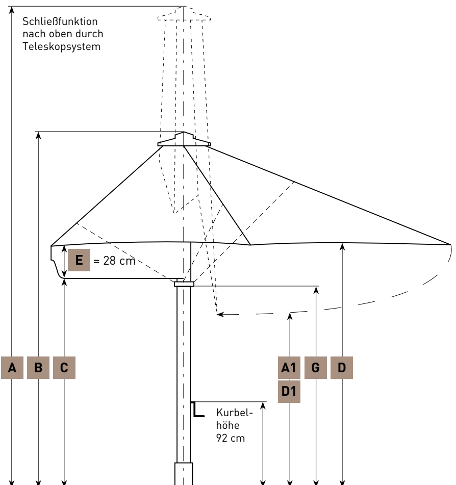
Seitenansicht A
